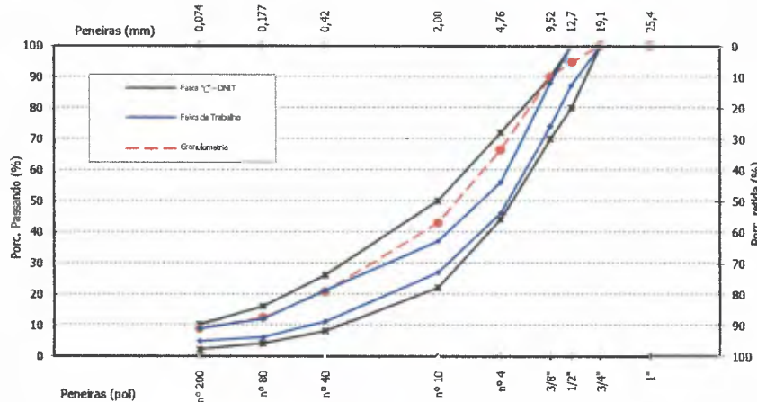
Gráfico da Análise Granulométrica
